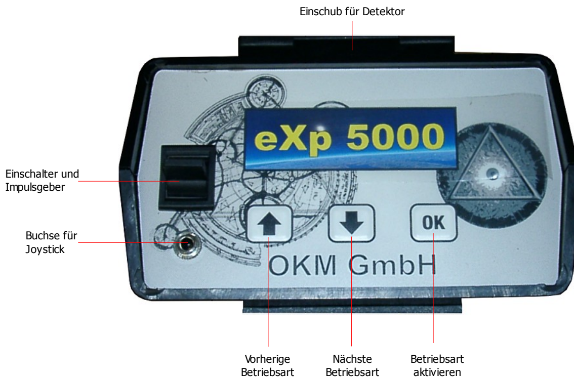
Abbildung 6.2: Kontrolleinheit, Vorderansicht
