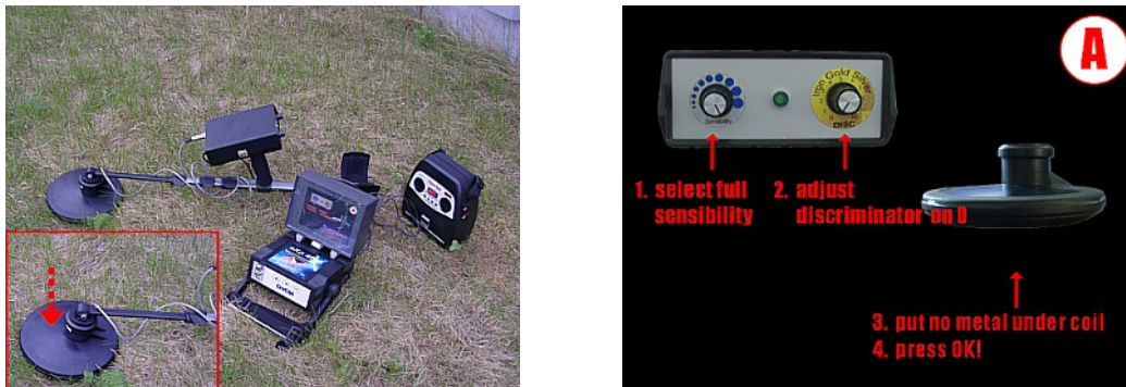
Abbildung 9.3: Kalibrierung des DDV-Systems, Schritt 1
