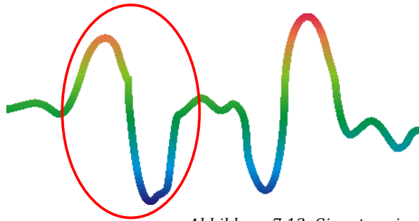
Abbildung 7.13: Signatur eines ferromagnetischen Metallobjekts
