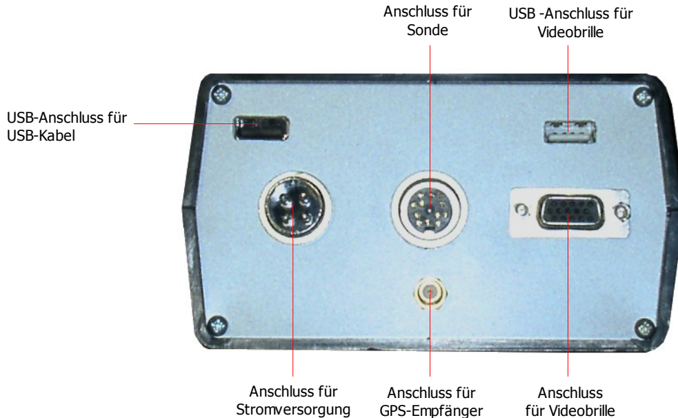
Abbildung 6.3: Kontrolleinheit, Rückseite
