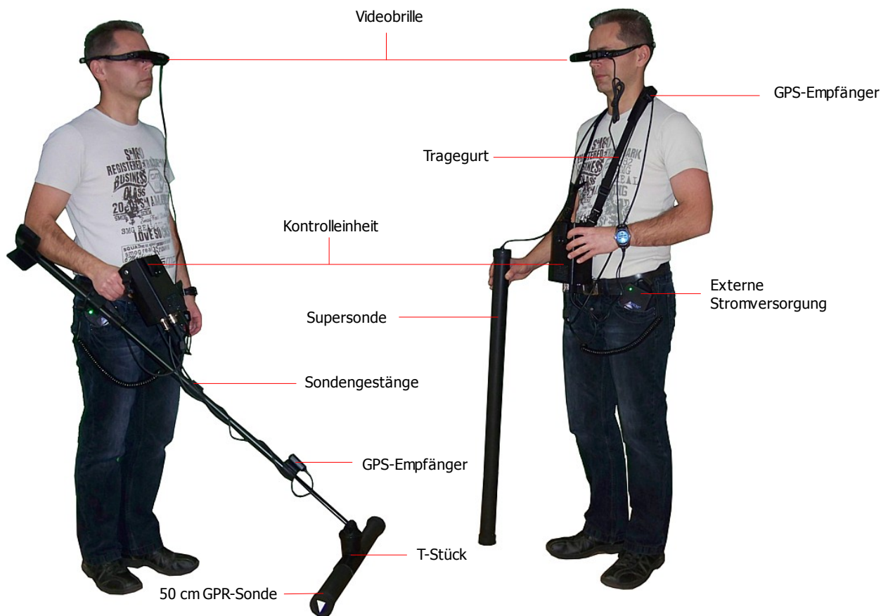
Abbildung 6.1: Kontrolleinheit mit Videobrille, Stromversorgung und Sonde
