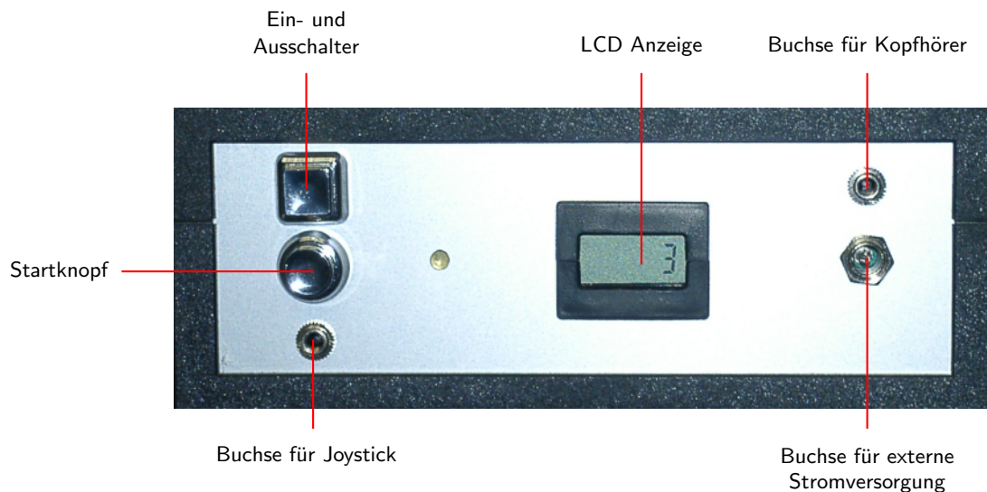
Abbildung 42: Vorderansicht
