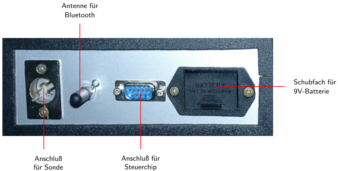
Abbildung 43: Rückseite
