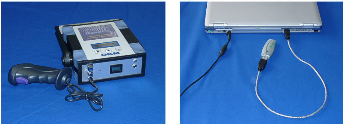
Abbildung 4: Anschluß des Joysticks und USB Dongle
